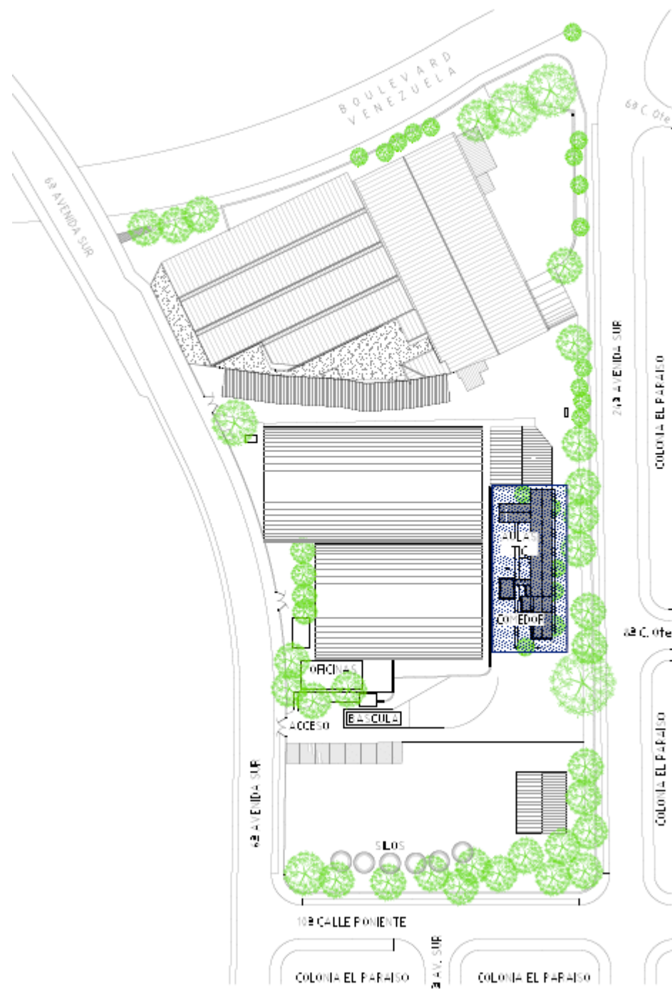
Esquema 3: Almacén Plantel El Paraíso, final 6ta calle Oriente #1105 Barrio San Esteban, San Salvador
